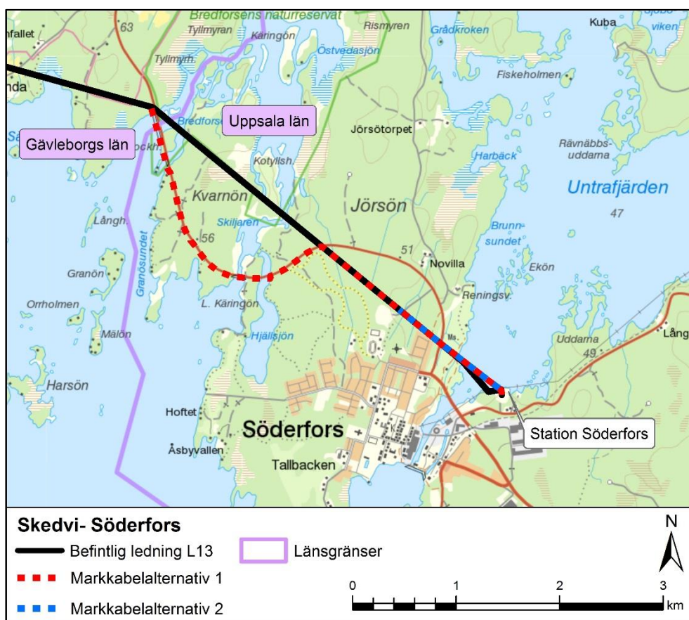
Karta över befintlig 130 kV kraftledning L13 genom Uppsala län.
