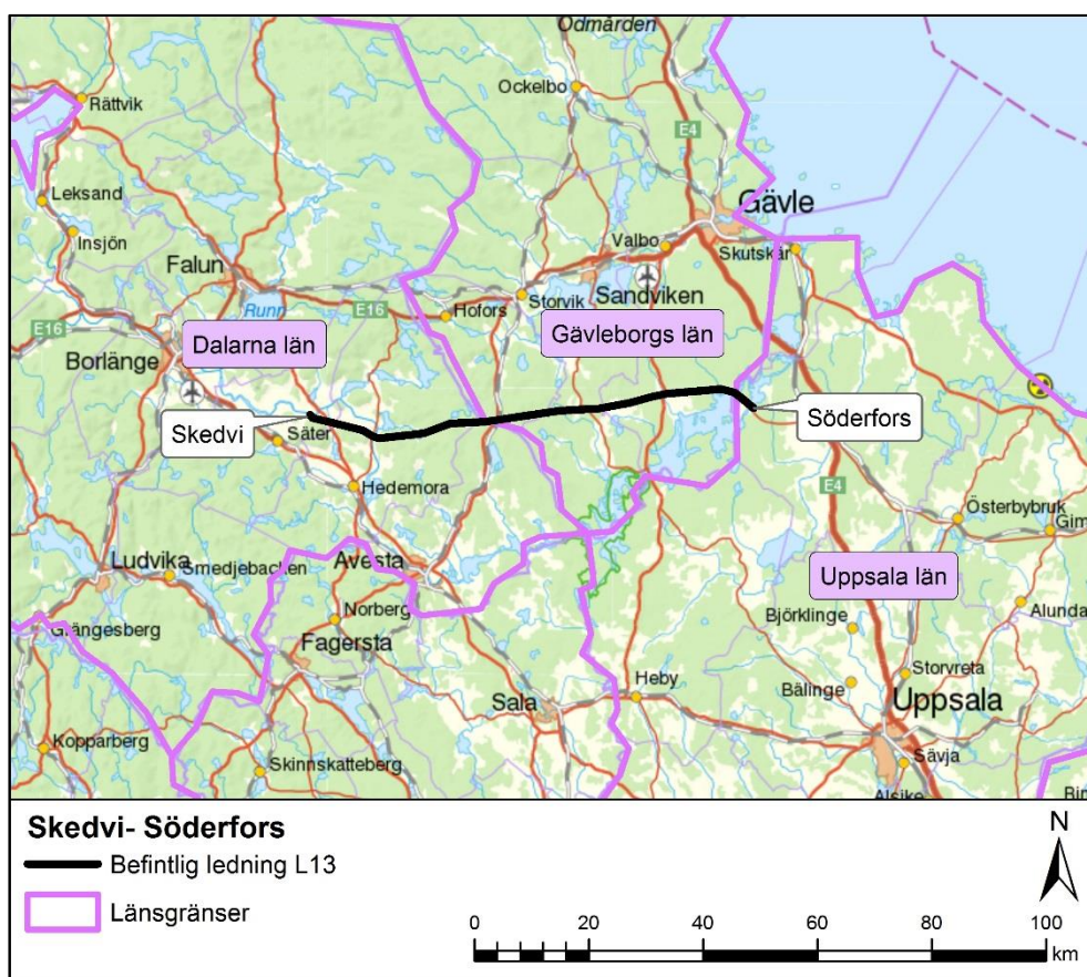
Karta över befintlig 130 kV kraftledning L13 genom Dalarnas, Gävleborgs och Uppsala län.
