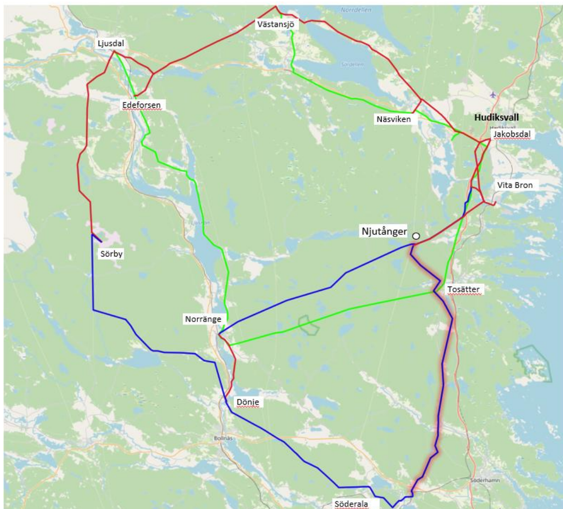
Figur 3. Mål bilden år 2032 för regionnätet i östra Hälsingland efter planerade åtgärder med nya stationer och ledningar. Blå linjer är nya eller ombyggda 130 kV ledningar.
