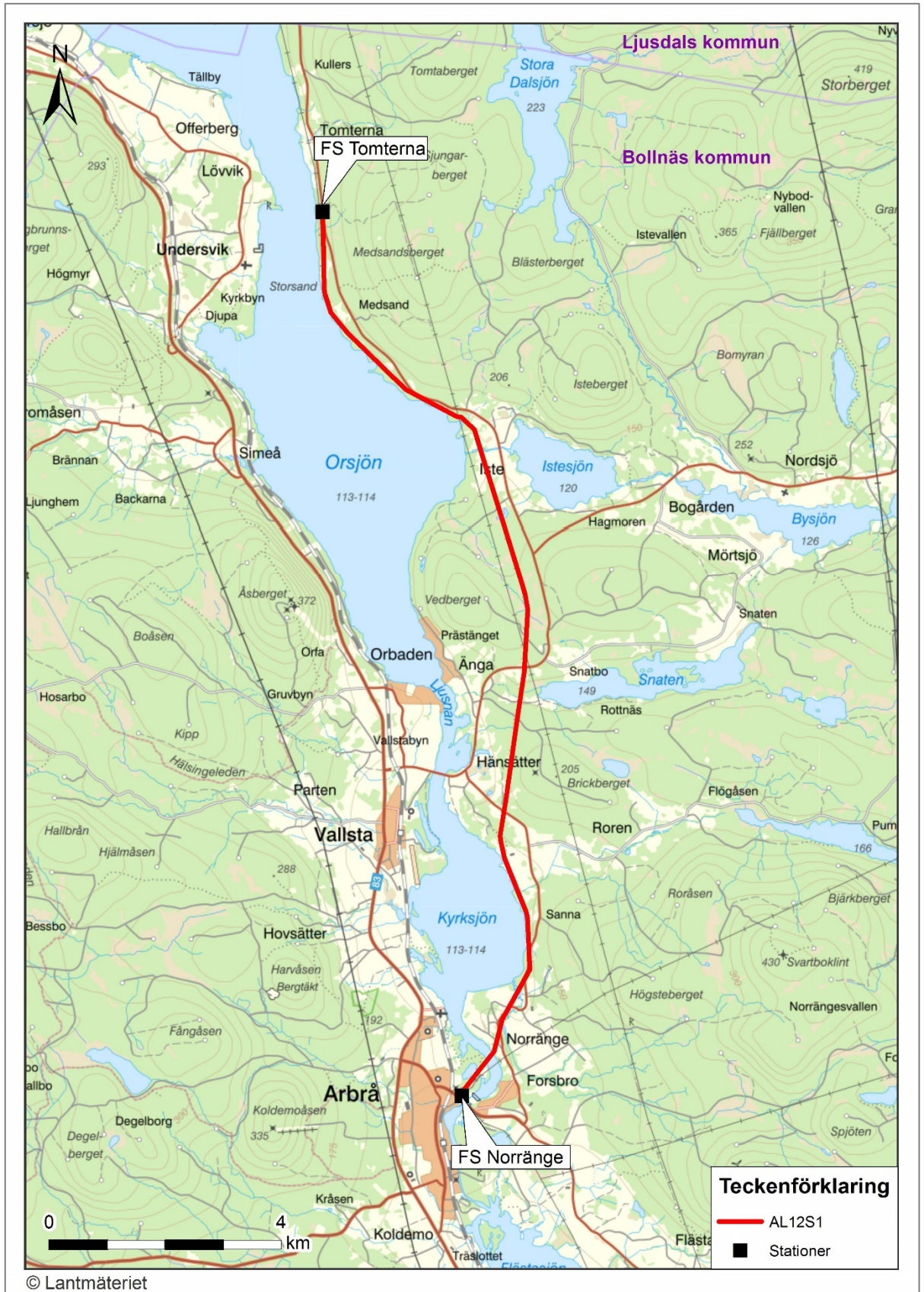
Figur 1. Översikt befintlig ledning, AL12S1, aktuell för förlängd koncession.
