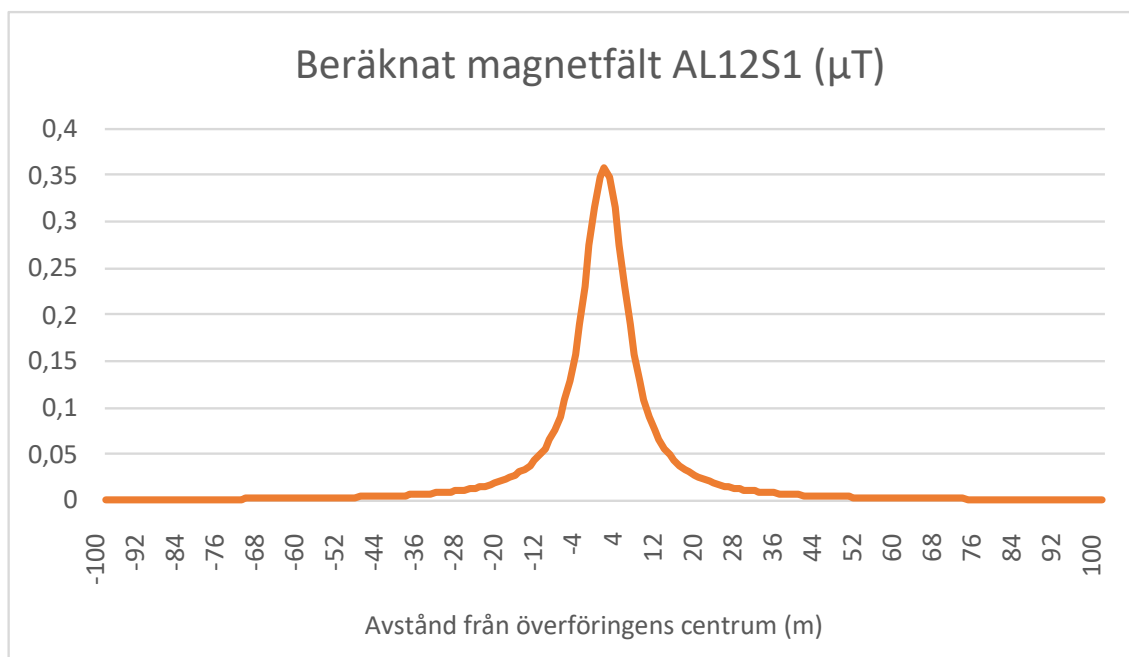
Figur 7. Beräknat magnetfält från befintlig luftledning AL12S1.
